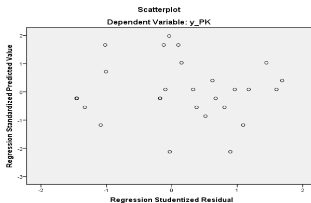
Gambar 2. Uji Heterokedastisitas
